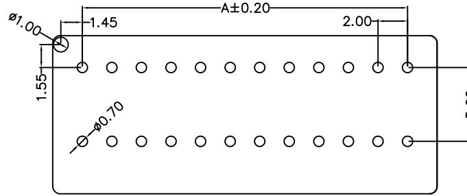
P.C.B LAYOUT
